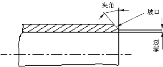
图 2 坡口示意图
